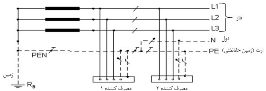
شکل پ-الف-۳- سامانه اتصال زمین TN-C-S
