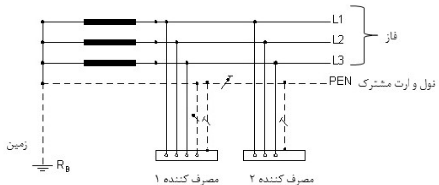
شکل پ-الف-۱- سامانه اتصال زمین TNC
