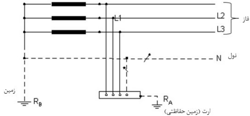
شکل پ-الف-۴: سامانه اتصال زمین TT
