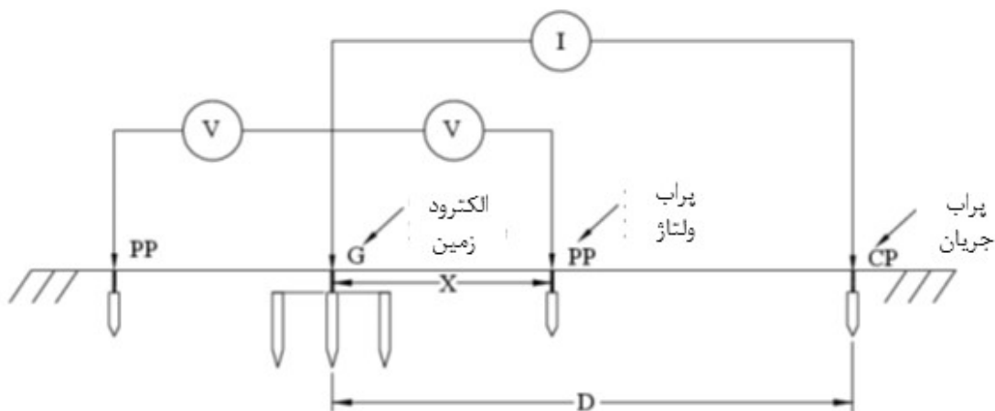
شکل پ-ت-۱- روش افت پتانسیل
