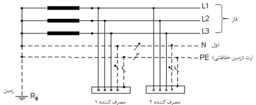
شکل پ-الف-۲-سامانه اتصال زمین TN-S
