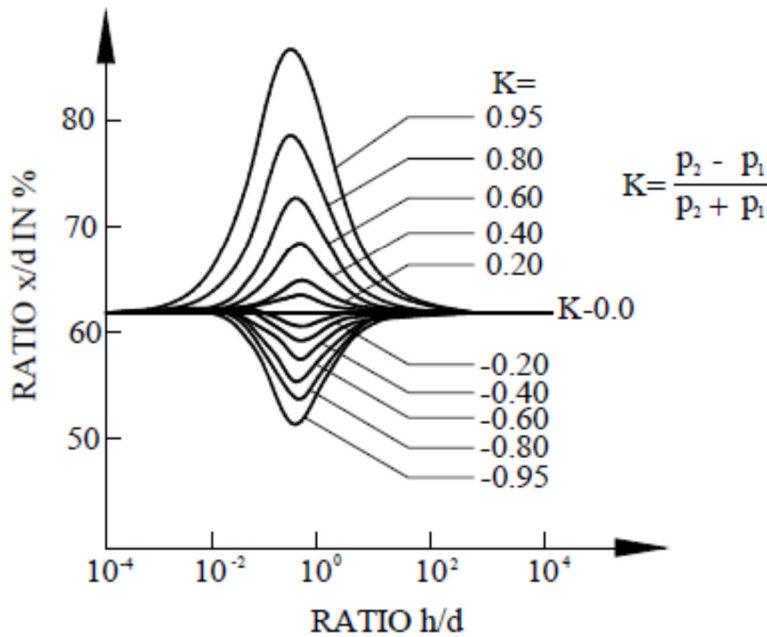
شکل پ-ت-۳- موقعیت مورد نیاز الکتروود ولتاژ در یک زمین دو لایه
