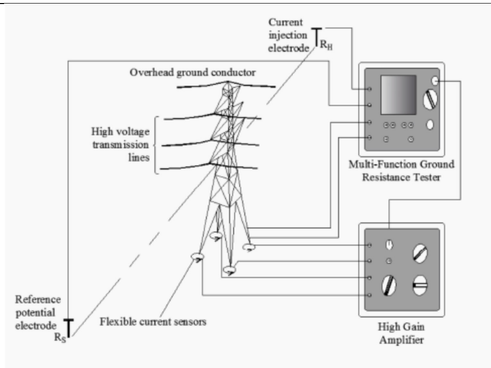
شکل پ-ت-۵- سامانه اندازه‌گیری مقاومت زمین دکل با استفاده از روش پتانسیل و اندازه‌گیری‌های جریان نشنی
