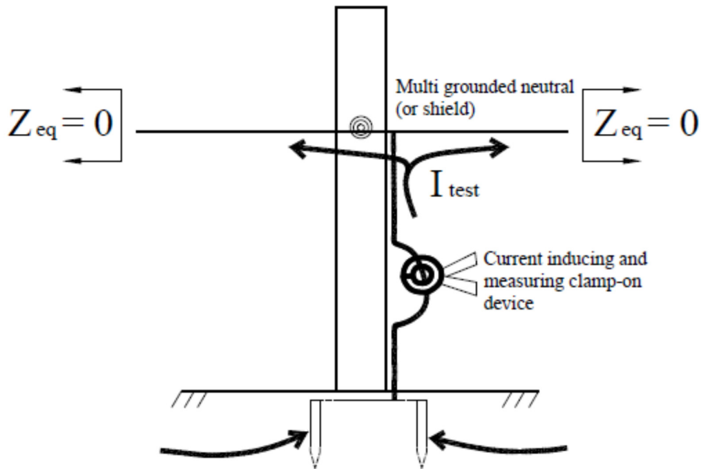
شکل پ-ت-۴- اندازه‌گیری مقاومت به روش کلمپی
