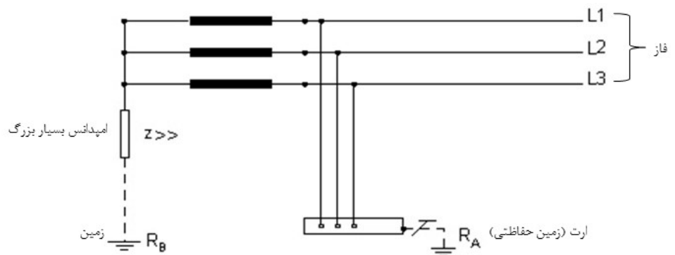
شکل پ-الف-۵: سامانه اتصال زمین IT
