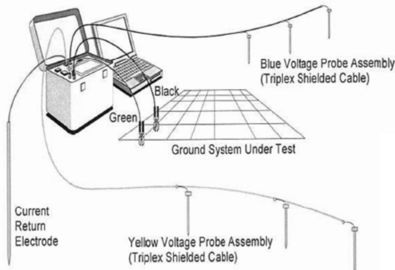
شکل پ-ت-۶- اندازه‌گیری امپدانس زمین با استفاده از مالتی متر زمین کامپیوتری
