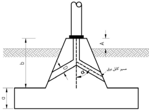
شکل ۱۳-۱۲: نمای نمونه فونداسیون بتنی پیش‌ساخته
