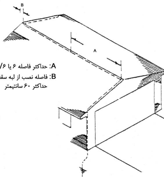
(الف) فواصل نصب بر روی خط‌الراس سقف‌های شیب‌دار
